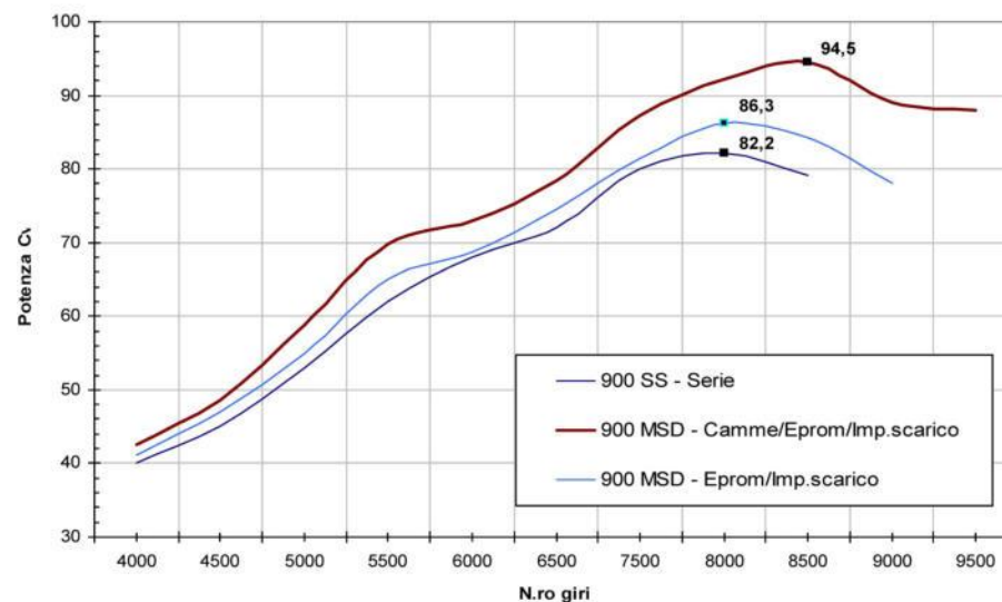
GRAFICO POTENZA MOTORE AL PIGNONE "SERIE DUCATI 900 - 2 VALVOLE" BANCO PROVA API
