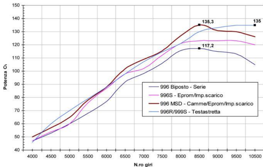
GRAFICO POTENZA MOTORE AL PIGNONE "SERIE DUCATI 996 - 4 VALVOLE" BANCO PROVA API
